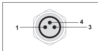
Schemazeichnung M8-Stecker
